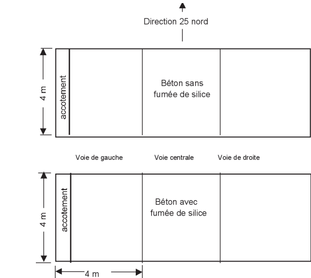
Figure 2 : Schéma de la planche d'essai de l'autoroute 25
