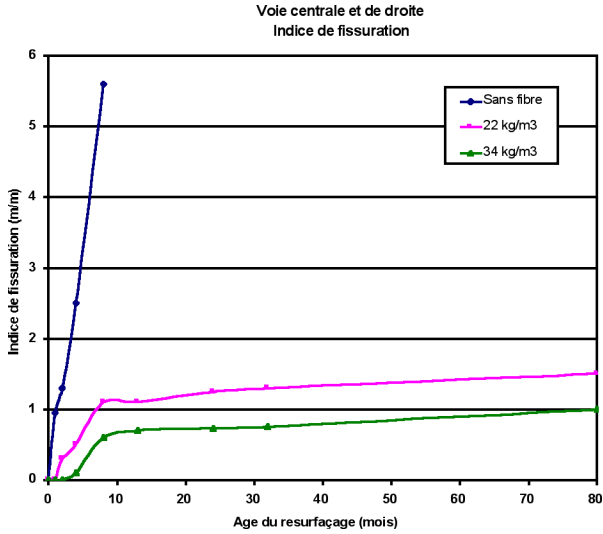
Figure 3 : Évolution de l'indice de fissuration moyen des resurfaçages en fonction du dosage en fibres (résultats basés uniquement sur le comportement de la voie centrale et de la voie de droite de l'autoroute 40)
