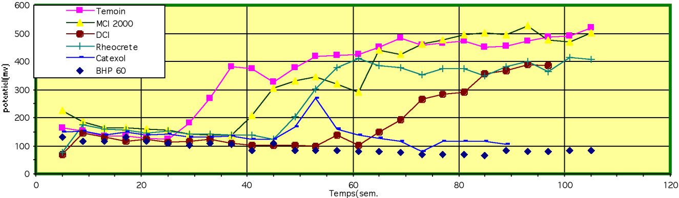
Figure 2 : potentiel de corrosion Cu/CuSO 4 100 semaines
