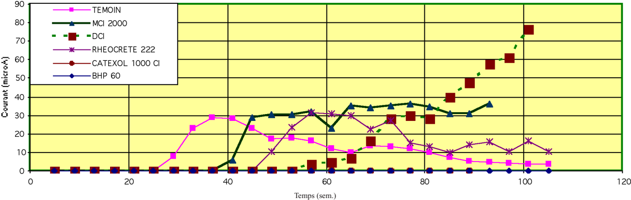
Figure 3 : courant de corrosion 100 semaines
