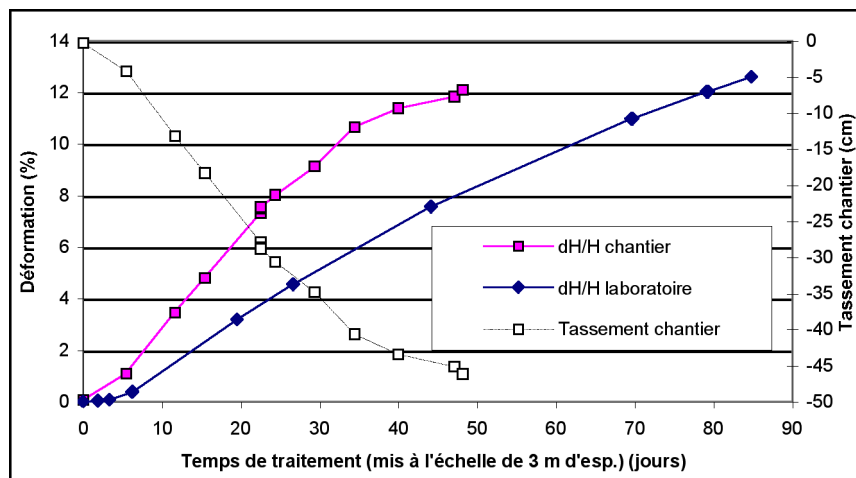
Figure 1 : Évolution du tassement et de la déformation dans le temps
