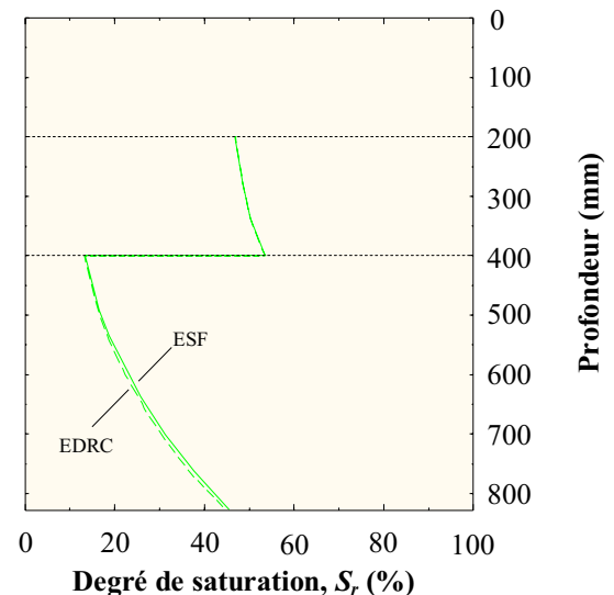
Figure 2 : Influence du système de drainage sur le degré de saturation sous la piste de roue externe en date du 3 mai
