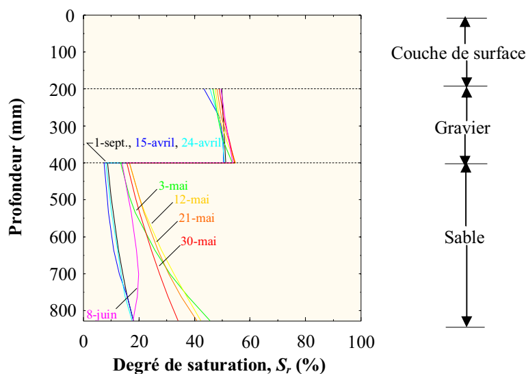
Figure 1 : Évolution temporelle du degré de saturation en piste de roue externe
