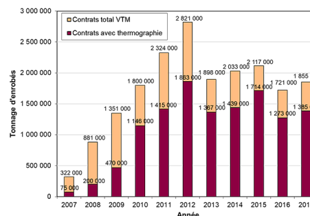
Figure 1 – Tonnage d'enrobés avec utilisation de la thermographie et d'un VTM
