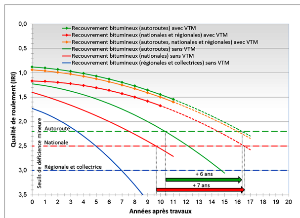
Figure 3 – Courbes d'évolution de la qualité de roulement pour les recouvrements bitumineux avec et sans VTM
