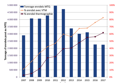
Figure 2 – Proportion des enrobés du MTQ posés avec la thermographie et/ou un VTM
